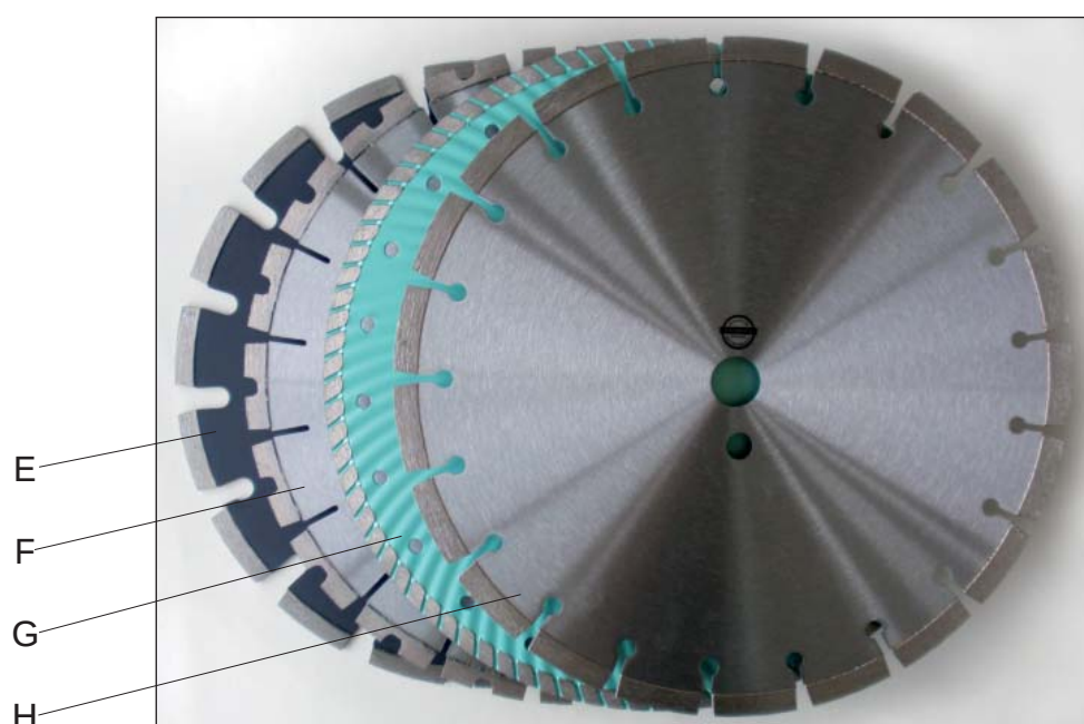
Diamantkapklinga (torrsågning) Laser/Sintrad
